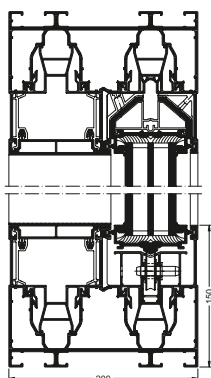
Вертикальное сечение Schüco ASS 77 PD.NI, масштаб 1:8 Vertical section detail Schüco ASS 77 PD.NI, scale 1:8
