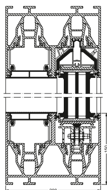
Вертикальное сечение Schüco ASS 77 PD.SI, масштаб 1:8 Vertical section detail Schüco ASS 77 PD.SI, scale 1:8
