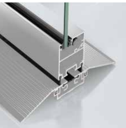
Вертикальное сечение ASS 50 FD.NI Vertical section detail of ASS 50 FD.NI
