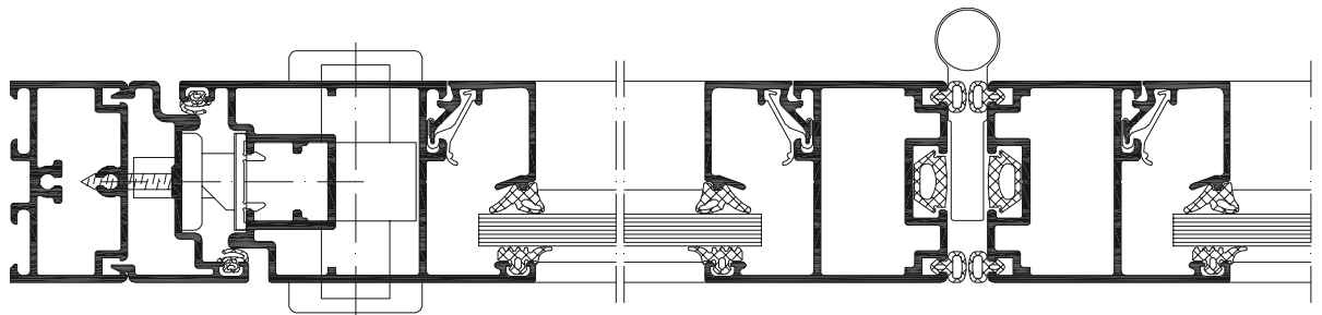
Schüco ASS 50 FD.NI, масштаб 1:2 Schüco ASS 50 FD.NI, scale 1:2
