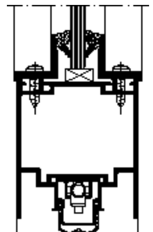
Вертикальное сечение, угловой штапик, масштаб 1:2 Vertical section detail, angled glazing bead, scale 1:2
